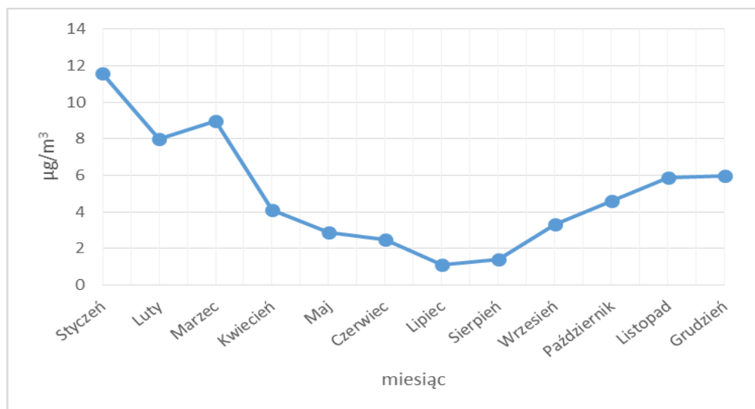
Rysunek 2 Średnioroczne stężenia benzenu w 2016 r., zaobserwowane na stacji pomiarowej w Czerwionce-Leszczynach przy ul. Kopalnianej
